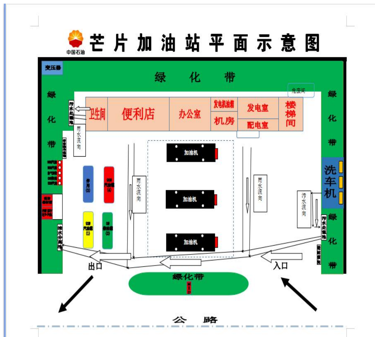
附图 2 总平面布置图及雨污分流图
