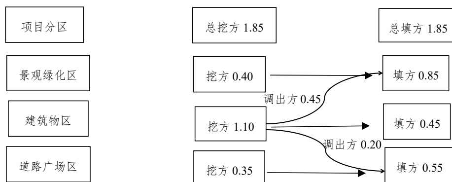
图 2.4-1 项目土石方平衡流向框图（单位：万 m 3 ）
