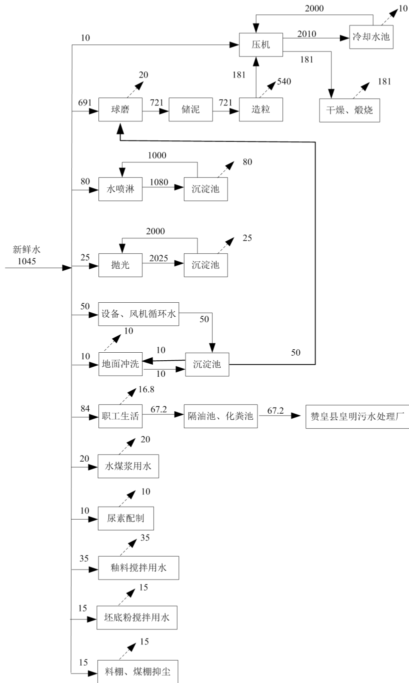
图 3-1 技改完成后全厂给排水平衡图 单位 (m 3 /d)
